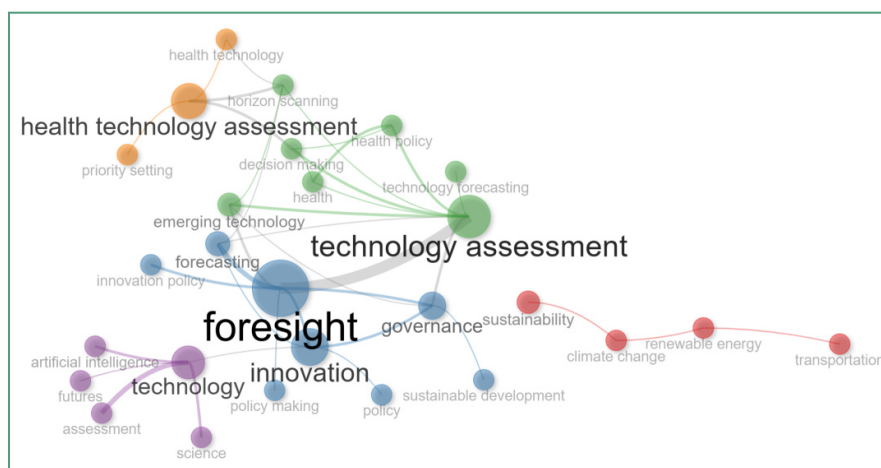
شکل ۲. شبکه هم‌واژگانی
